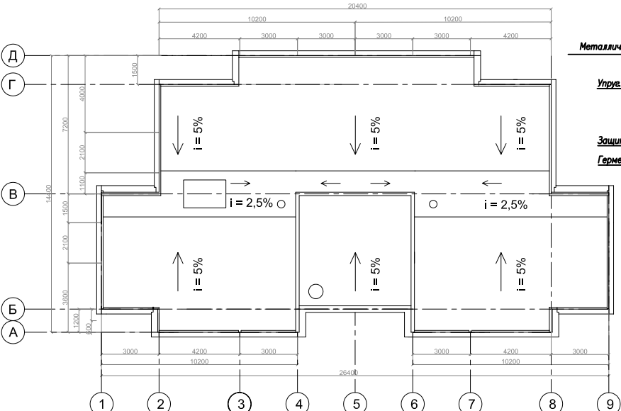
План кровли
