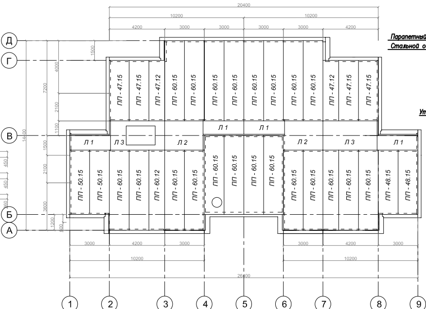
План кровли
