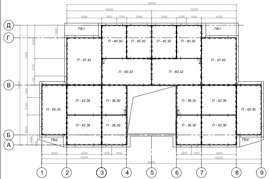
План перекрытия
