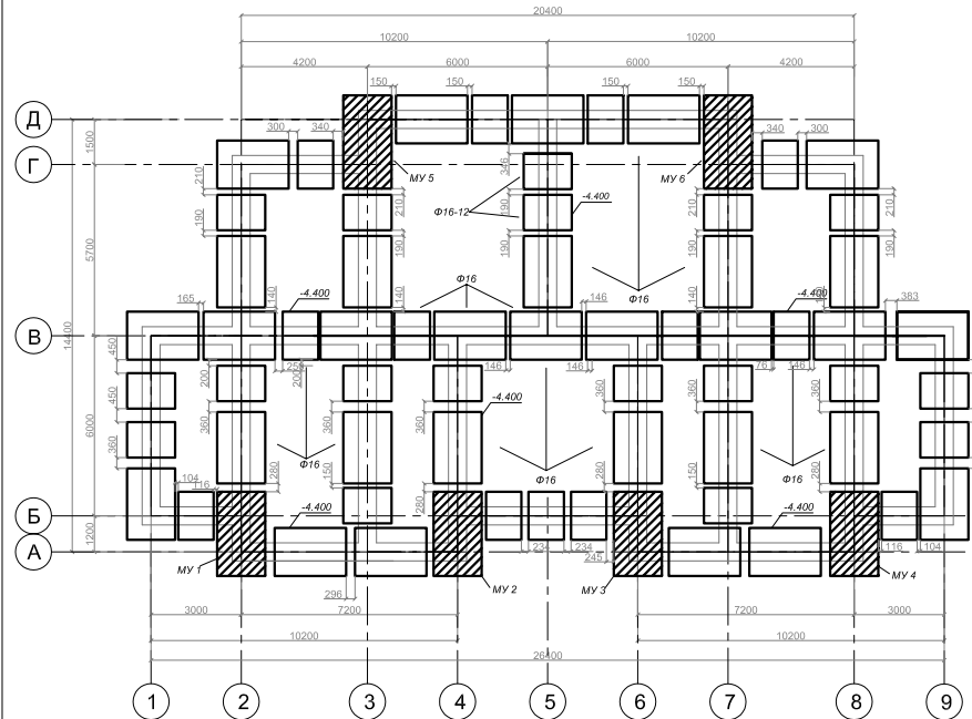
План перекрытия
