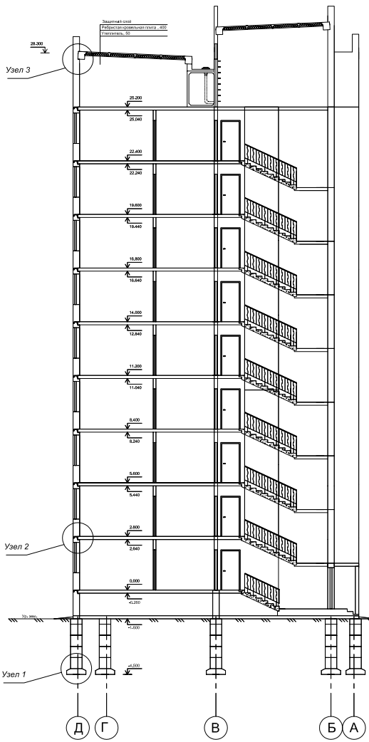
Разрез Е - А
